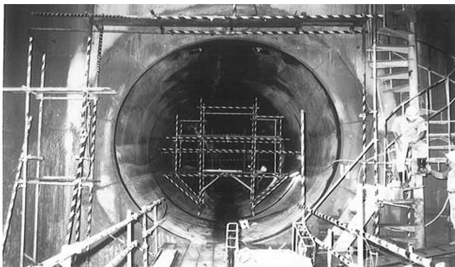
(北多摩一号処理区関連区域【小川幹線】) 昭和56年8月撮影
