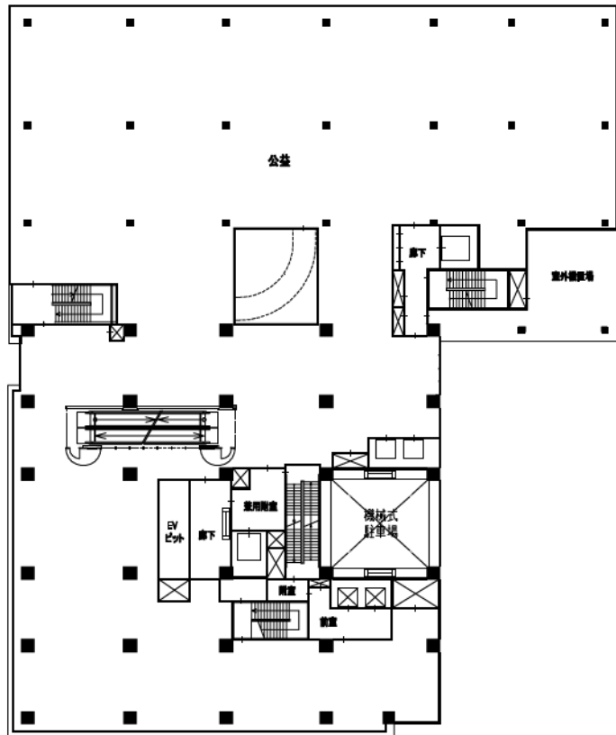
4階平面図
