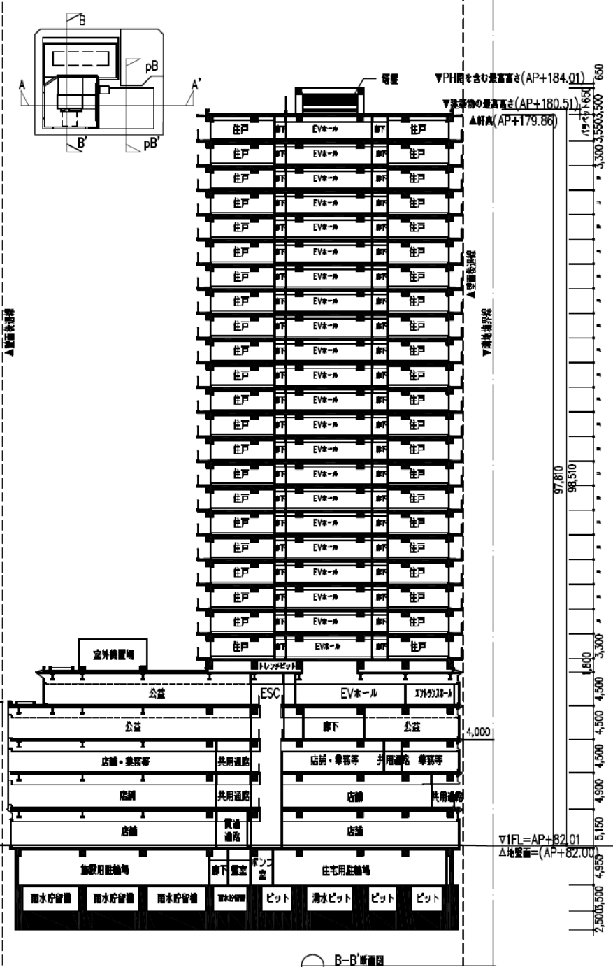
(4) 施設建築物の設計図 断面図 1/500
